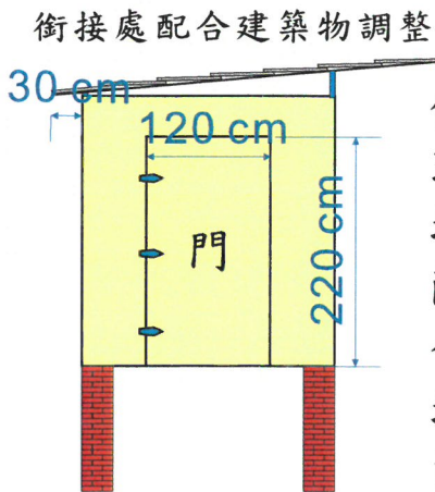
正視圖
