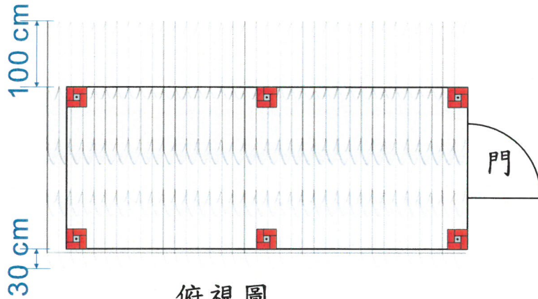
俯視圖
