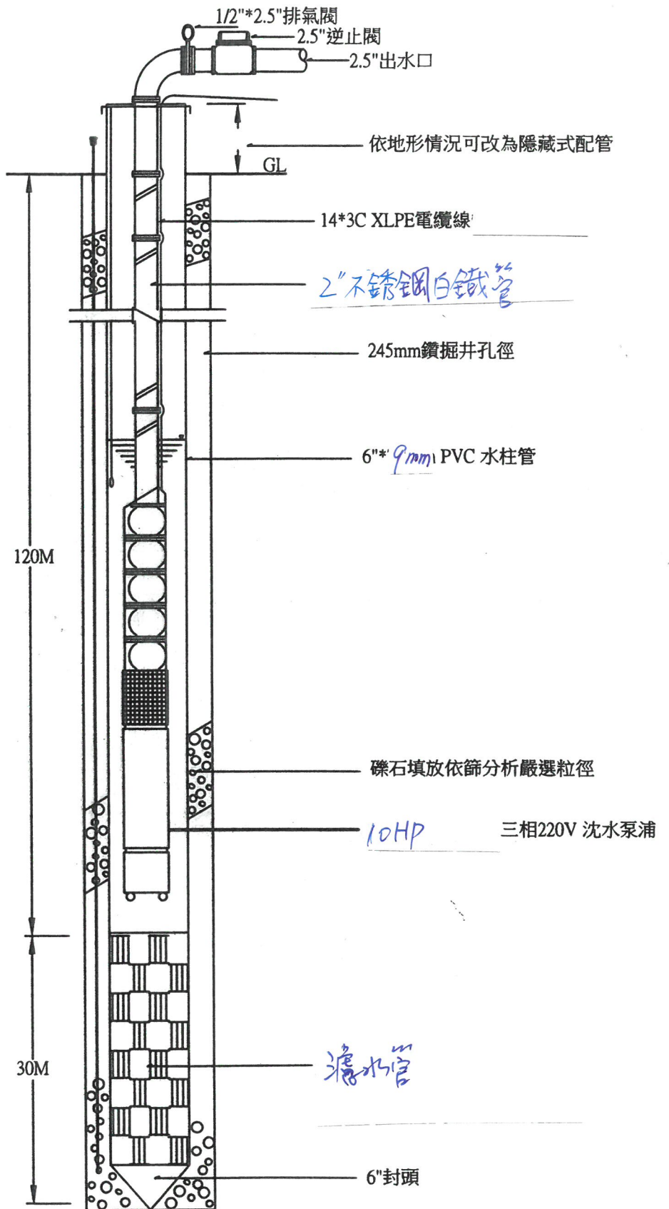
烏來文山農場150M水井詳圖
